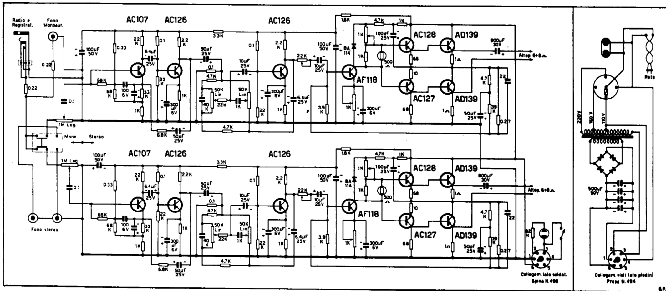
Geloso G251HF Amplifier
